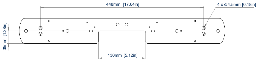
VOORAANZICHT
