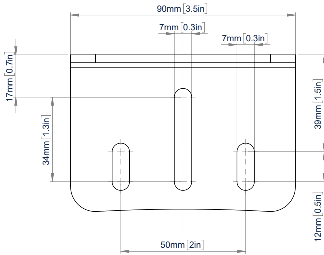
BOVENAANZICHT
