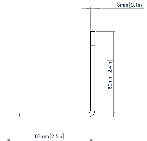
ZIJAAANZICHT
