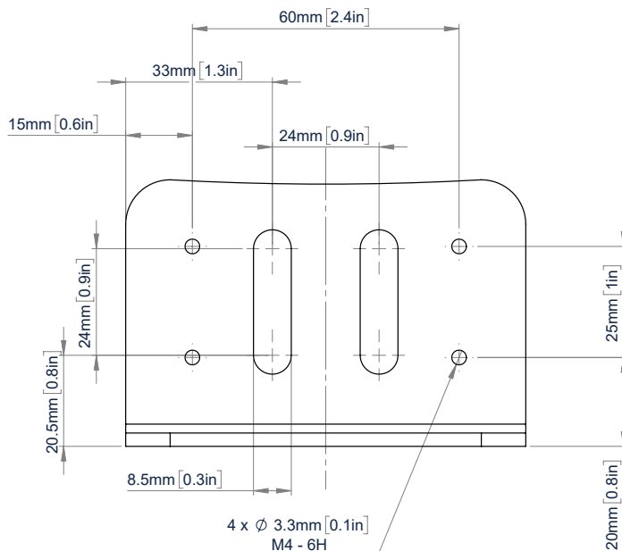
VOORAANZICHT
