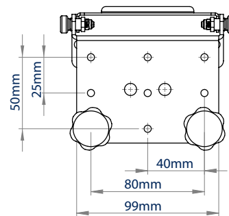
ACHTERAANZICHT
