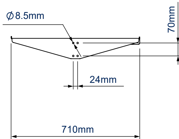
ACHTERAANZICHT
