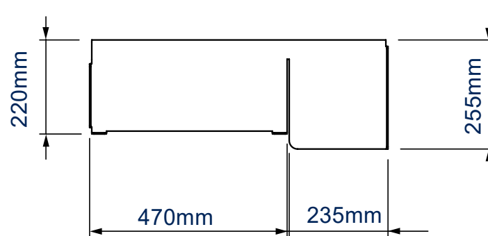
BOVENAANZICHT
