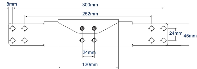
VOORAANZICHT
