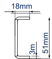
ZIJAAANZICHT
