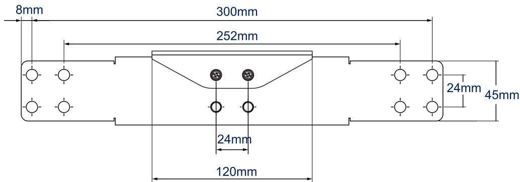
VOORAANZICHT
