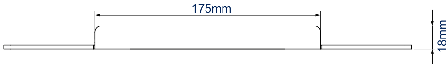
BOVENAANZICHT
