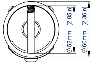
BOVENAANZICHT
