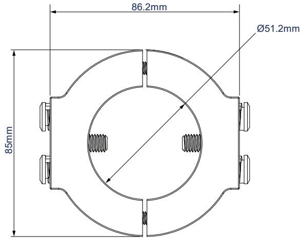
BOVENAANZICHT
