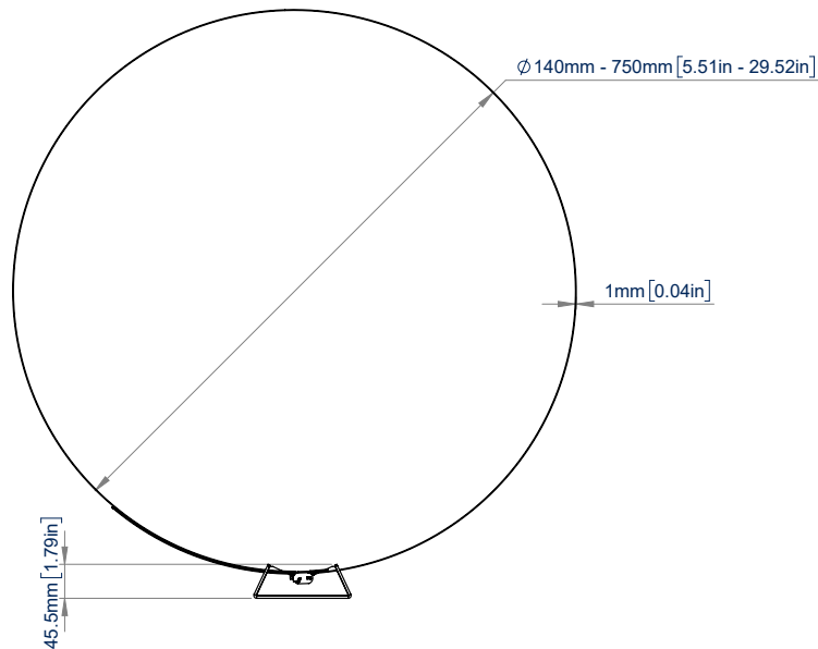
BOVENAANZICHT
