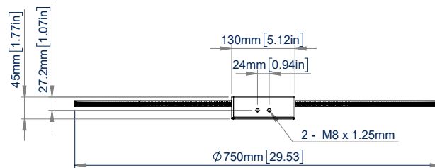
VOORAANZICHT
