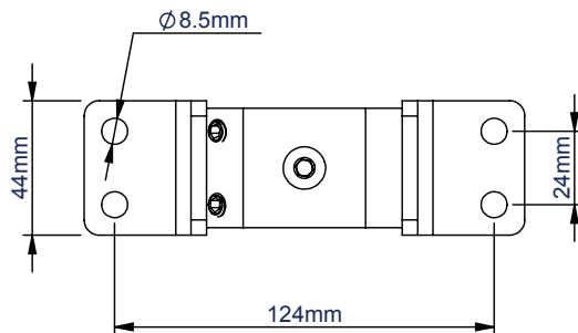
ACHTERAANZICHT
