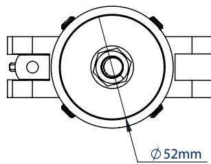
BOVENAANZICHT
