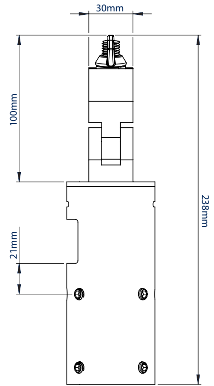
ZIJAAANZICHT
