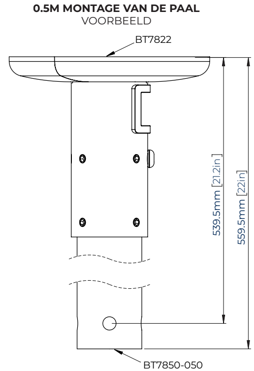
ZIJAAANZICHT
