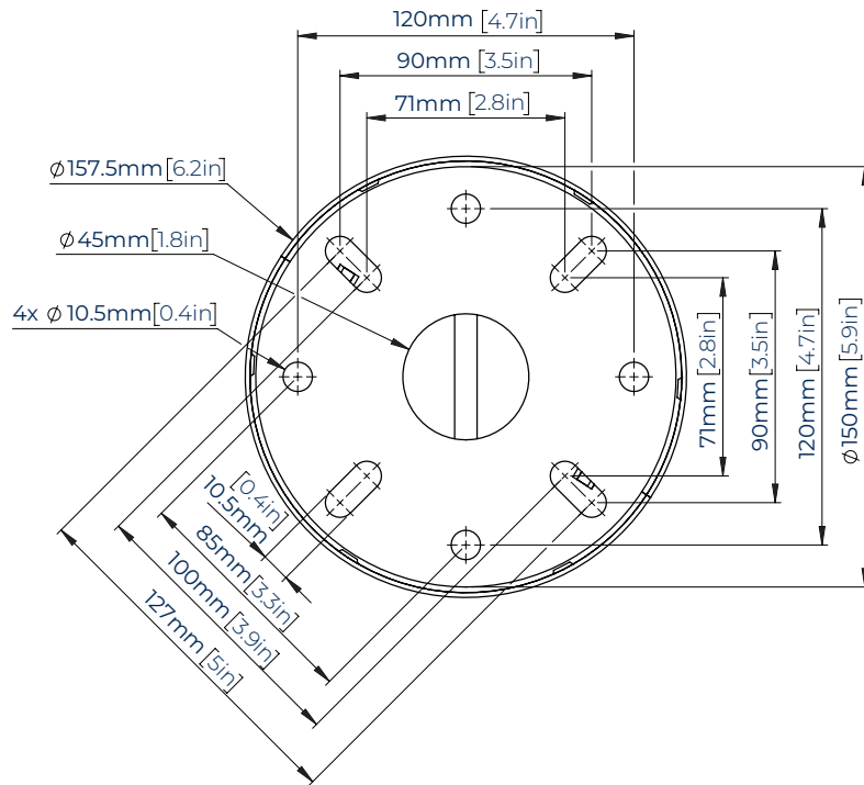
BOVENAANZICHT
