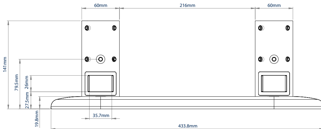
ZIJZICHT MET AFDEKPLAAT
