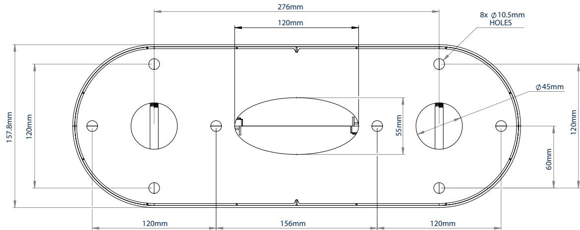
BOVENAANZICHT MET AFDEKPLAAT
