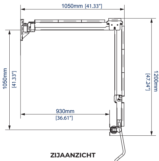
ZIJAANZICHT – MAXIMALE UITSCHUIFLENGTE
