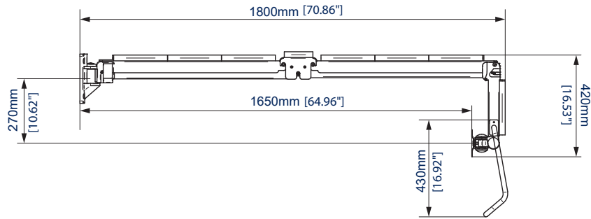
ZIJAANZICHT – MAXIMALE UITSCHUIFLENGTE
