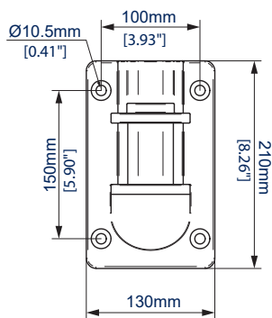
WANDPLAAT
