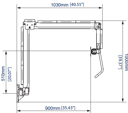
ZIJAANZICHT
