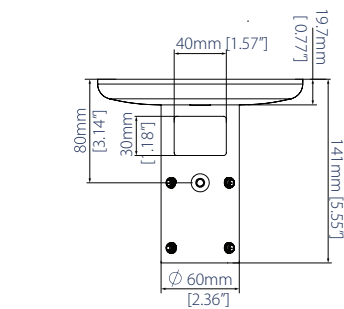
PLAFONDPLAAT - ACHTERAANZICHT
