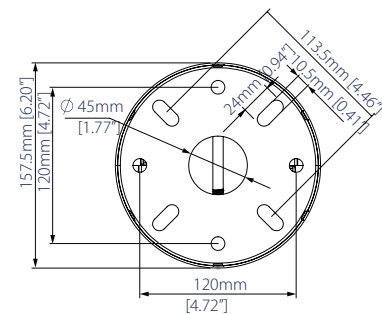
PLAFONDPLAAT - BOVENAANZICHT
