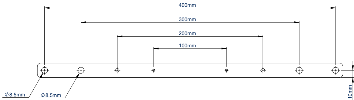
BOVENAANZICHT
