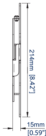
ZIJAAANZICHT WANDPLAAT & INTERFACEPLAAT
