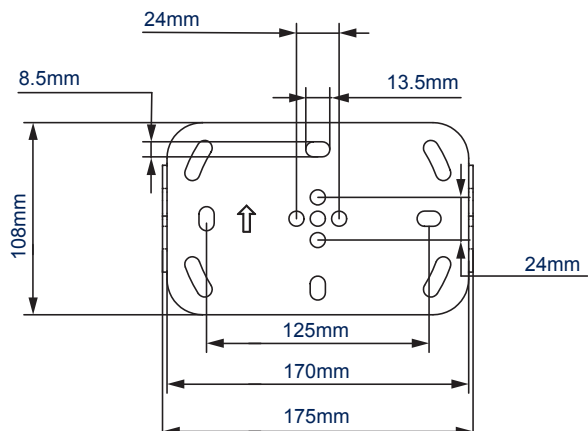
WANDPLAAT VOORAANZICHT
