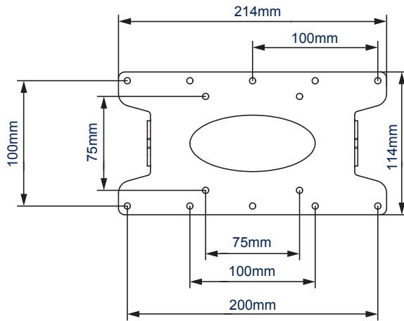
AANSLUITPLAAT VOORAANZICHT
