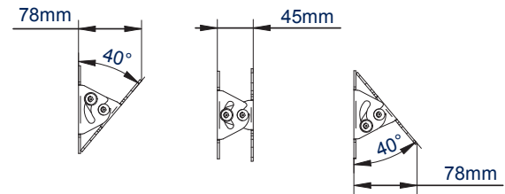
ZIJZICHT ZONDER ADAPTERARMS
