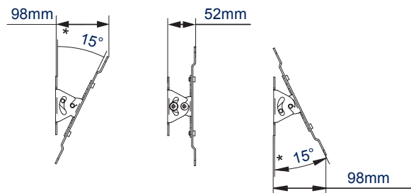
ZIJZICHT MET ADAPTERARMEN
