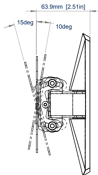
ZIJAANZICHT
