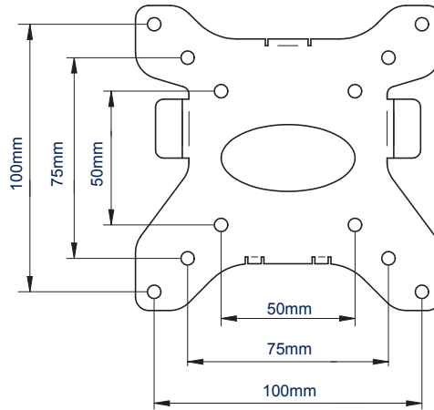
VOORAANZICHT AANSLUITPLAAT
