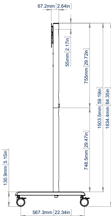
ZIJAANZICHT
