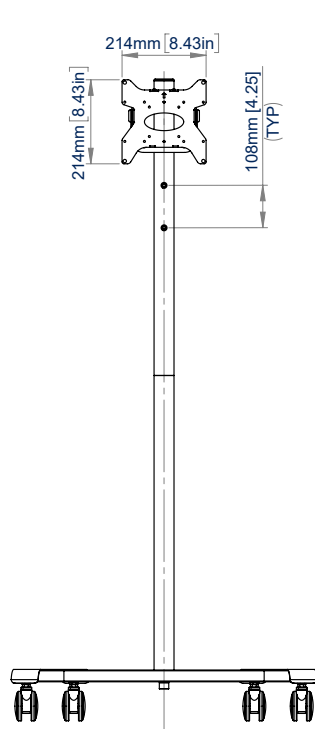
VOORAANZICHT
