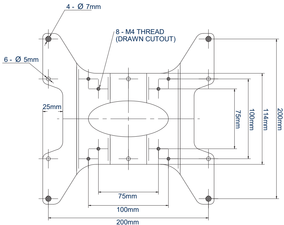
VOORAANZICHT
