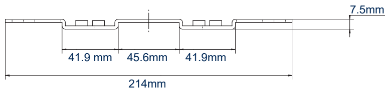
ZIJAANZICHT
