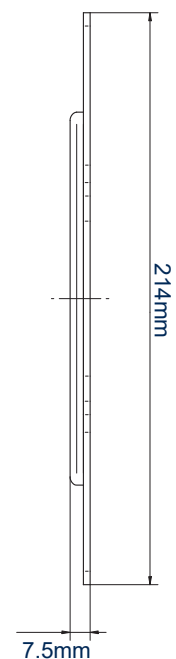
ZIJAANZICHT
