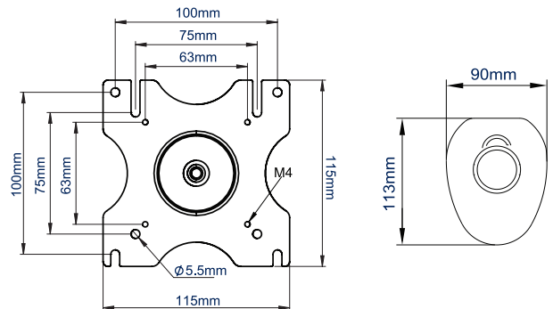
VOORAANZICHT INTERFACE
