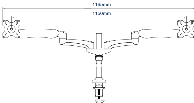
VOORAANZICHT
