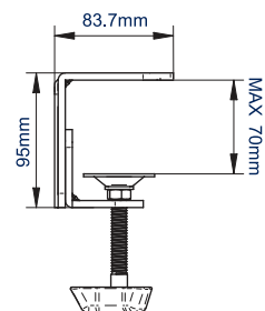
ZIJZICHT BUREAUKLEM
