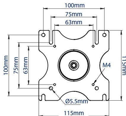
VOORAANZICHT - INTERFACE
