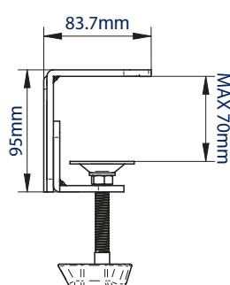
ZIJZICHT - BUREAUKLEM
