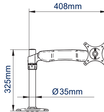
VOORAANZICHT
