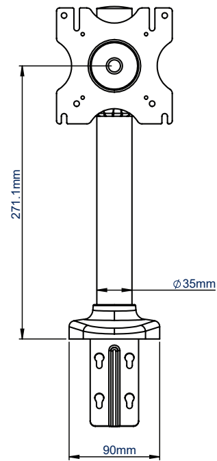
VOORAANZICHT
