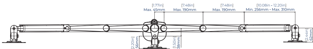
BOVENAANZICHT
