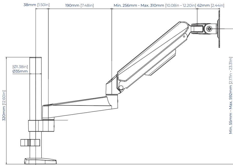
ZIJZICHT
