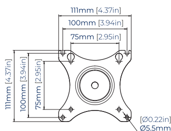
AANSLUITPLAAT
