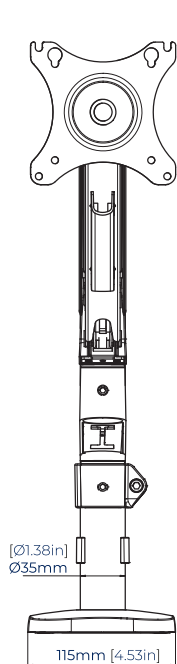
VOORAANZICHT
