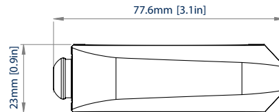
VISTA LATERAL CON PLACA DE CUBIERTA
