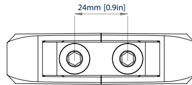
VISTA FRONTAL CON PLACA DE CUBIERTA
