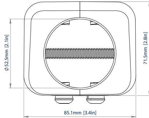
VISTA SUPERIOR CON PLACA DE CUBIERTA
