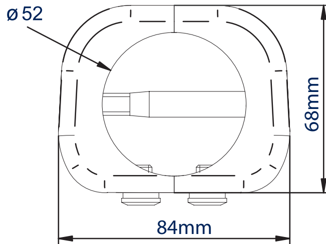
BOVENAANZICHT
