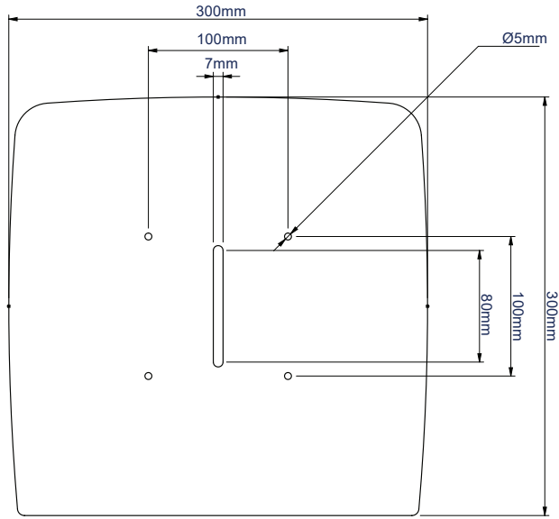
BOVENAANZICHT
