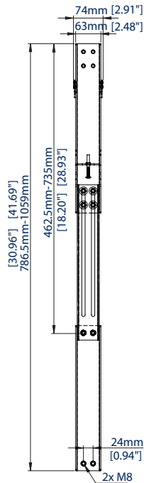
VOORAANZICHT ONDER HET SCHERM UITGEBREID
