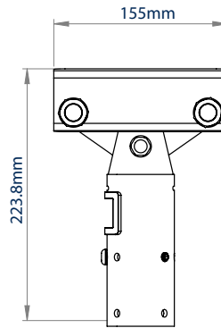
ZIJAAANZICHT
