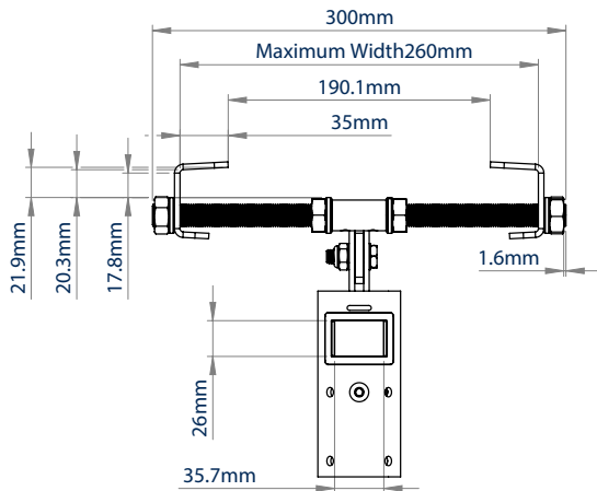
VOORAANZICHT MAXIMALE BREEDTE
