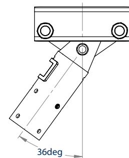
KANTELVERSTELLING 36 GRADEN (MAXIMAAL)
