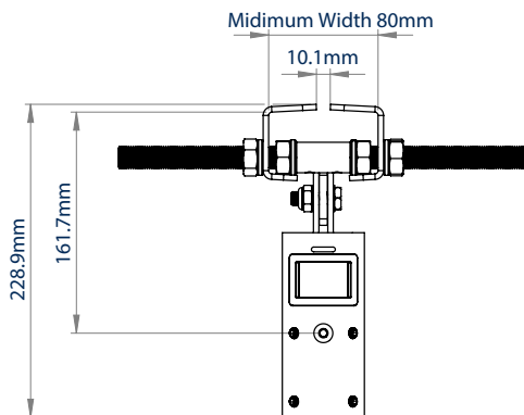
VOORAANZICHT MINIMALE BREEDTE
