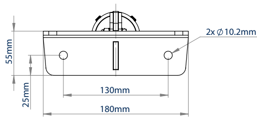
BOVENAANZICHT
