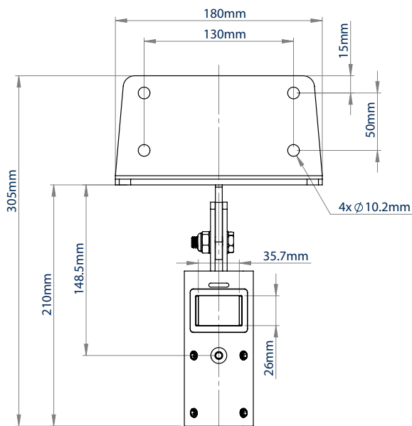
ACHTERKANT
