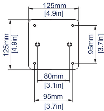
BOVENSTE PLAAT
