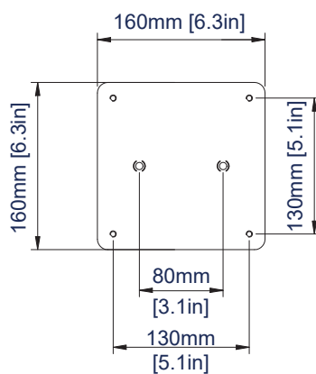
BOVENSTE PLAAT
