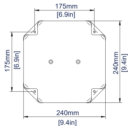
BASISPLAAT
