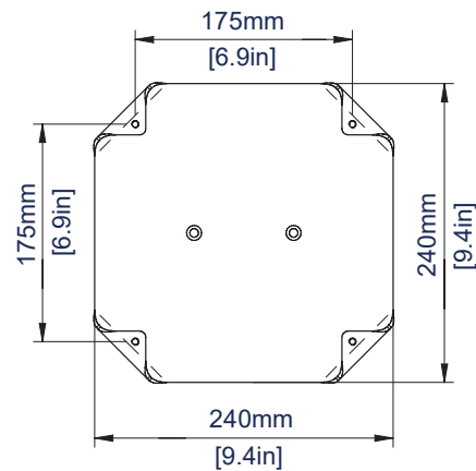
BASISPLAAT
