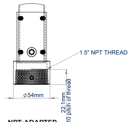
NPT-ADAPTER VOORAANZICHT
