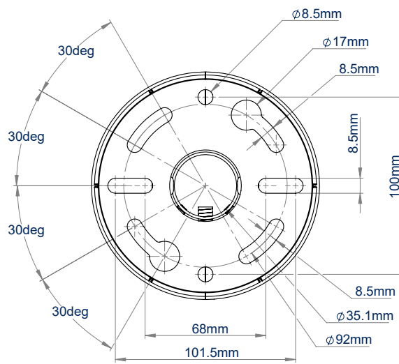
BT5965-FD100 VOORAANZICHT
