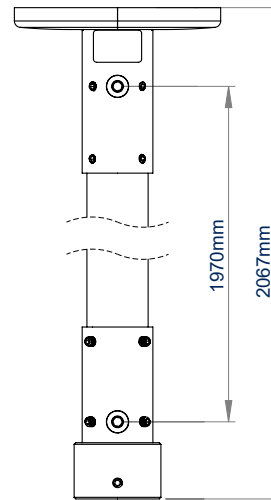
BT5965-FD200 VOORAANZICHT
