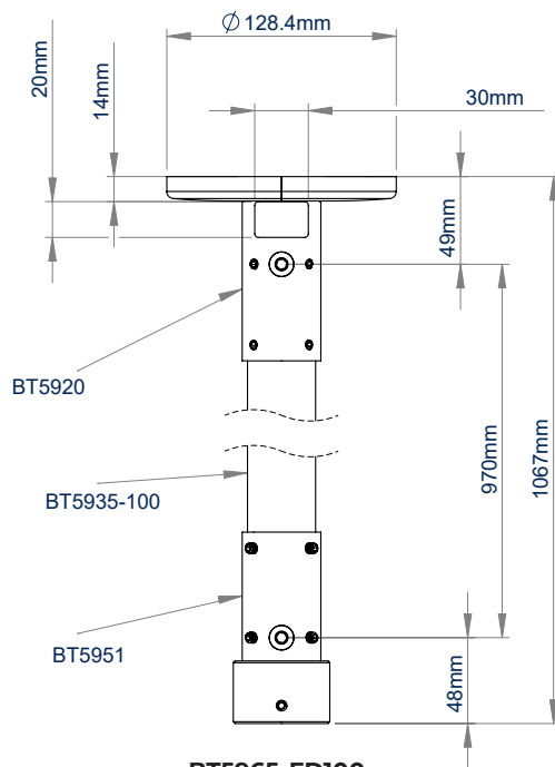
BT5965-FD100 VOORAANZICHT
