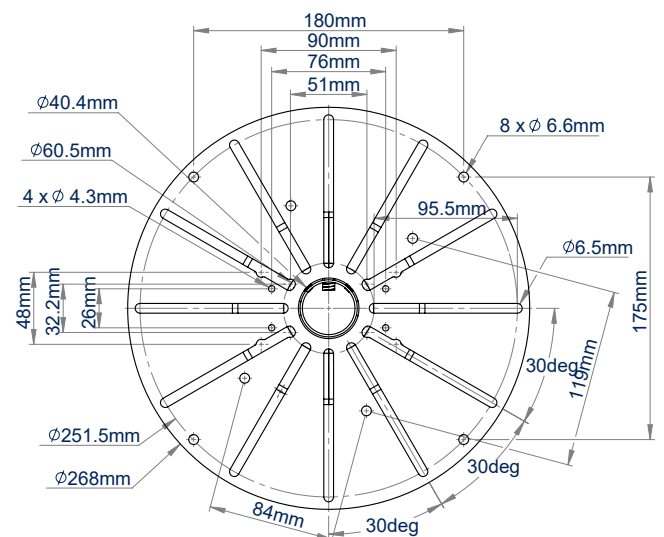
BEVESTIGING VOOR BEWAKINGSCAMERA ONDERZICHT
