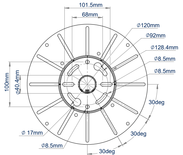
PLAFONDPLAAT BOVENAANZICHT
