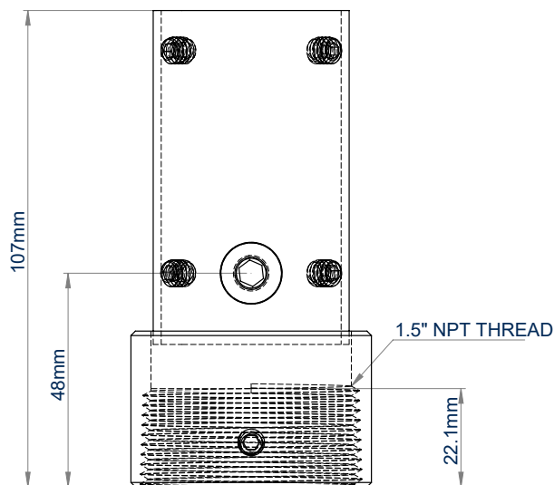
VOORAANZICHT
