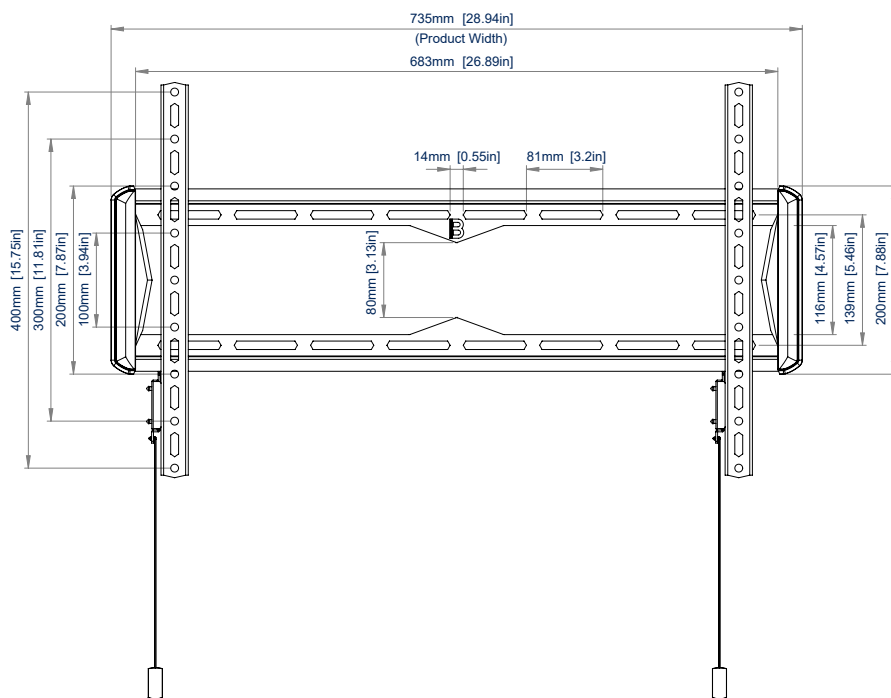
VOORAANZICHT
