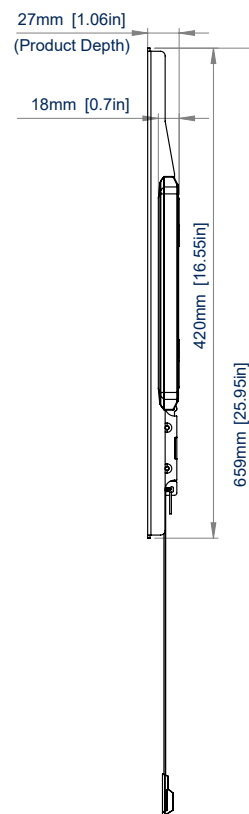
ZIJAAANZICHT
