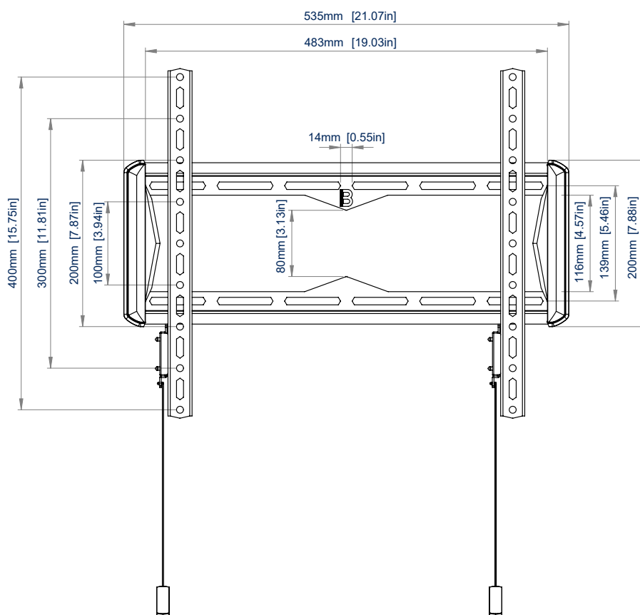
VOORAANZICHT
