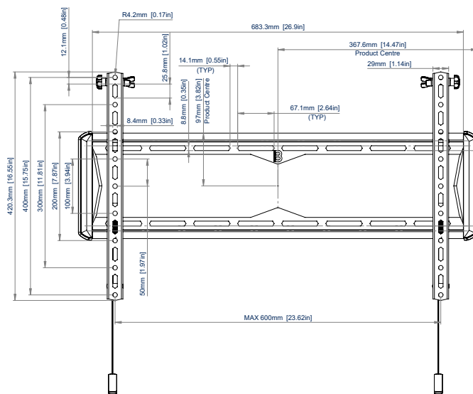
VOORAANZICHT
