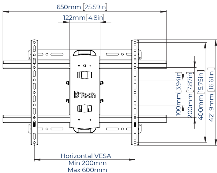
VOORAANZICHT
