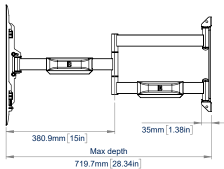
ZIJZICHT WITH EXTENSION
