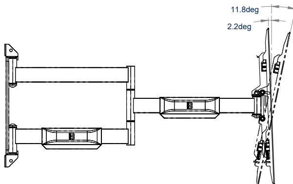
ZIJZICHT MET KANTELFUNCTIE
