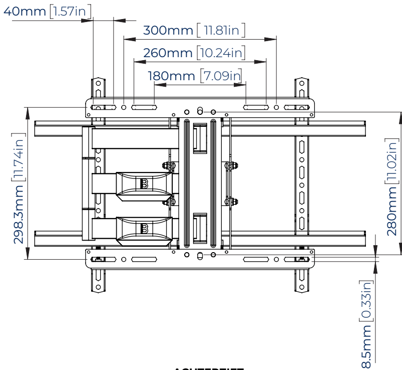
ACHTERZIJT
