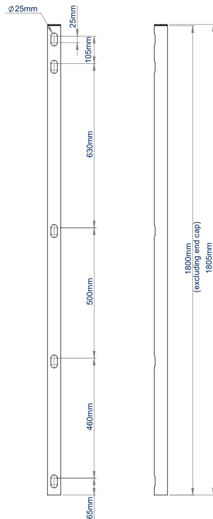
ACHTERZICHT
