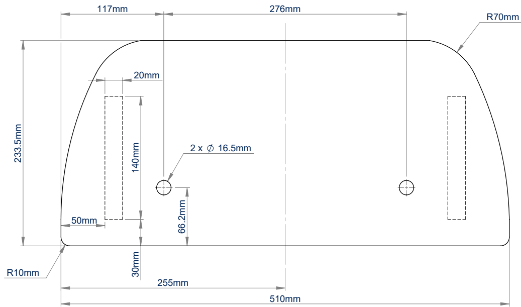
BOVENAANZICHT
