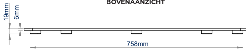
VOORAANZICHT
