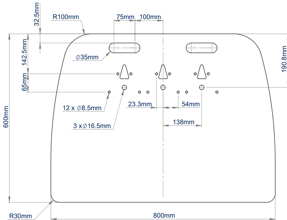
BOVENAANZICHT
