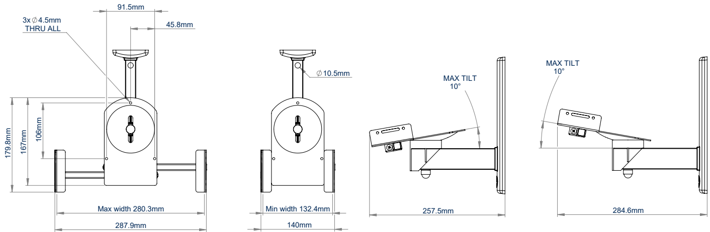
BOVENAANZICHT
